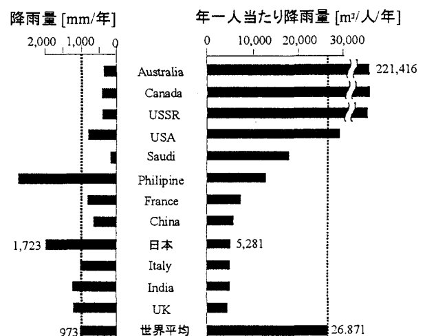
図1 平均降水量と一人当たり降雨量 2)
