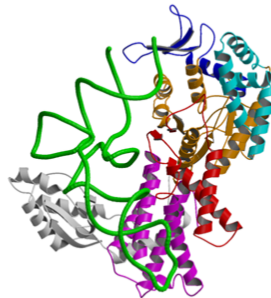
P. holkoshii 由来アルギニル-tRNA酵素とtRNAの複合体
