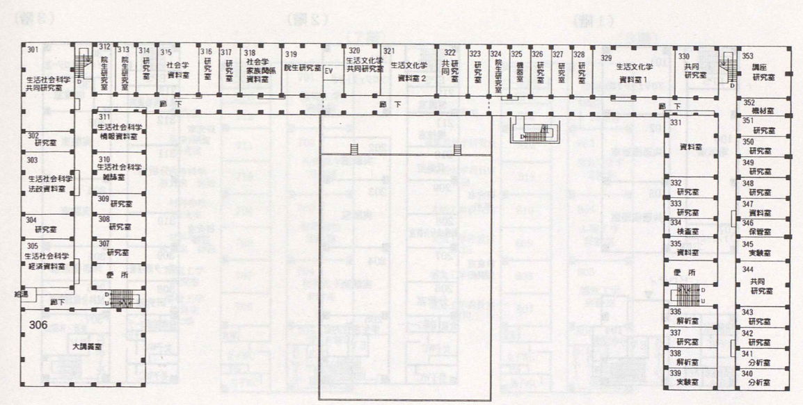
3階
