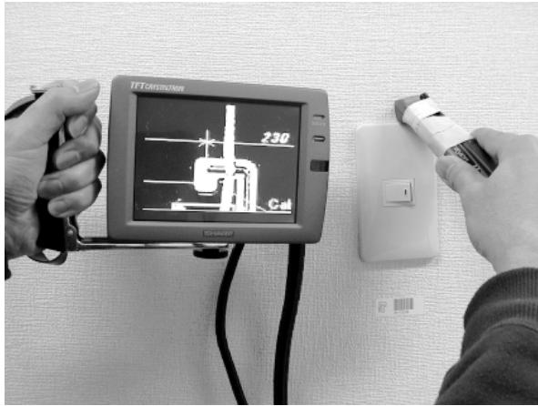
図1. Scroll Browserの全景。LCDと指示装置部で構成される。指示装置を壁に当てて動かすと、その場所の情報がLCDに表示される。
