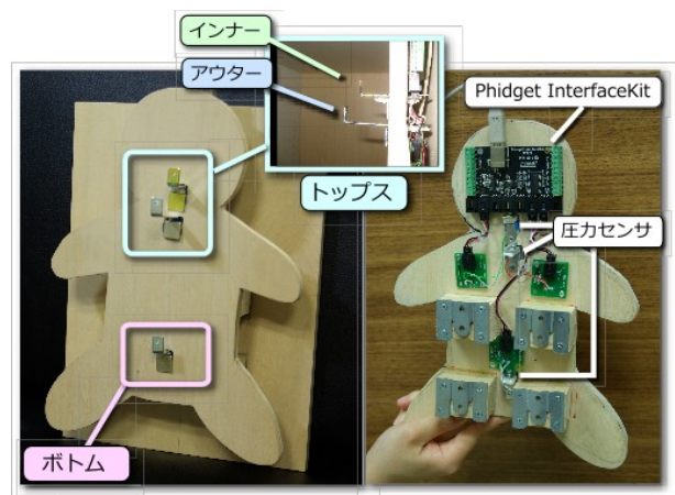
図 2: フックセンサのプロトタイプ。
